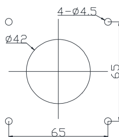
安装F型手柄 门板开孔尺寸
