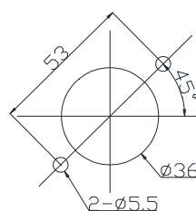
安装A型手柄 门板开孔尺寸
