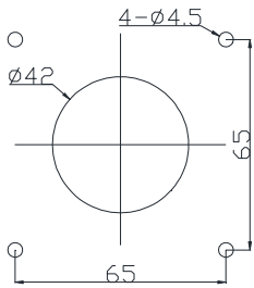
安装F型手柄 门板开孔尺寸
