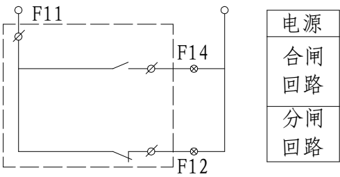
辅助触头接线图
